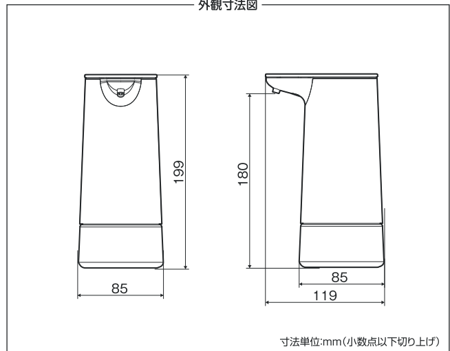
寸法単位:mm(小数点以下切り上げ)
